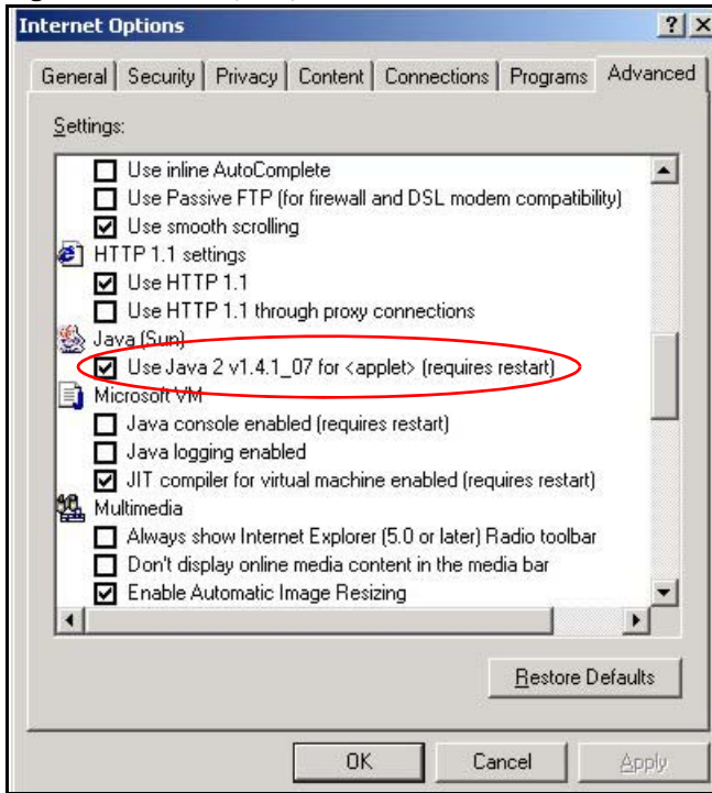
Figure 190 Java (Sun)
