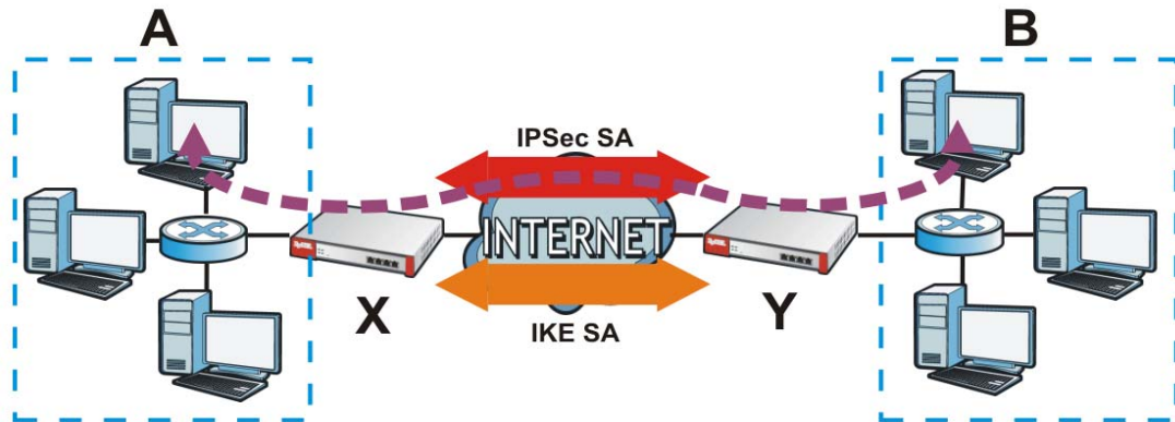
Figure 228 VPN: IKE SA and IPsec SA
